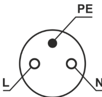
Rysunek 1: Układ wyprowadzeń gniazda zasilającego
